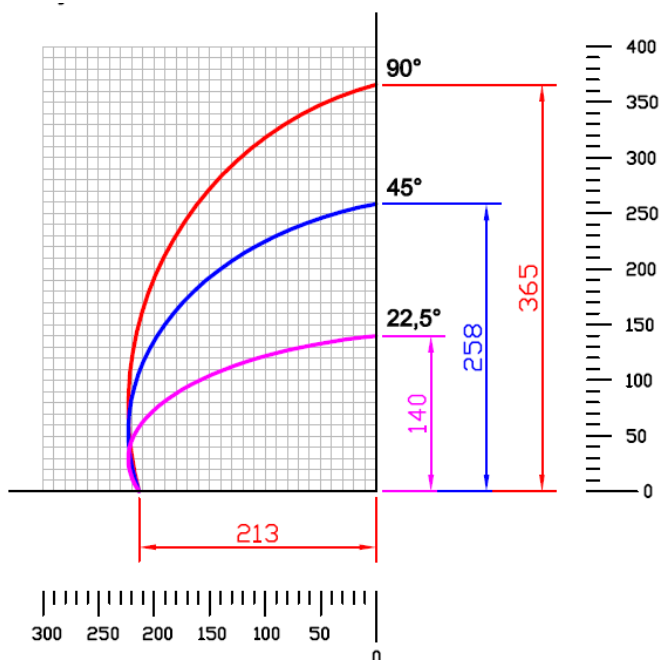
Diagramma di taglio con lama Ø600
