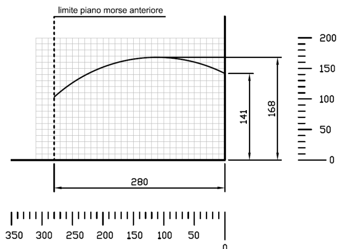
Diagramma di taglio troncatrice Retta con lama \varnothing 500 mm (tolleranza \pm 3 mm)
